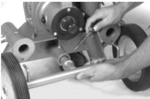
图3 — 从32型小车上拆下滚沟机
