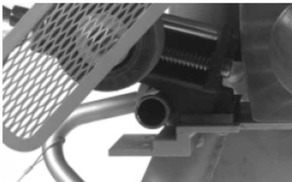
图12A — 2"-16"位置
